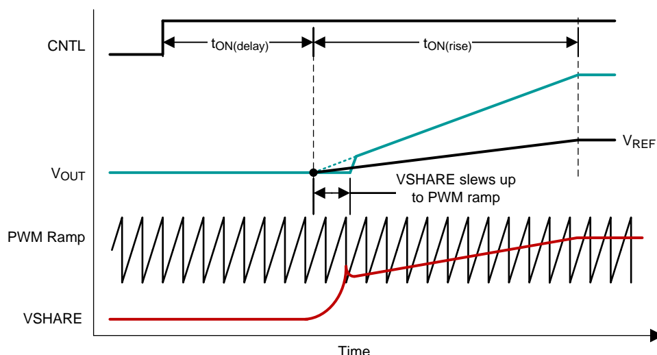
图 31. Soft-Start Timing
