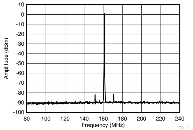
图 6-9. 156.25 ± 78.125-MHz HCSL Differential Output Spectrum
