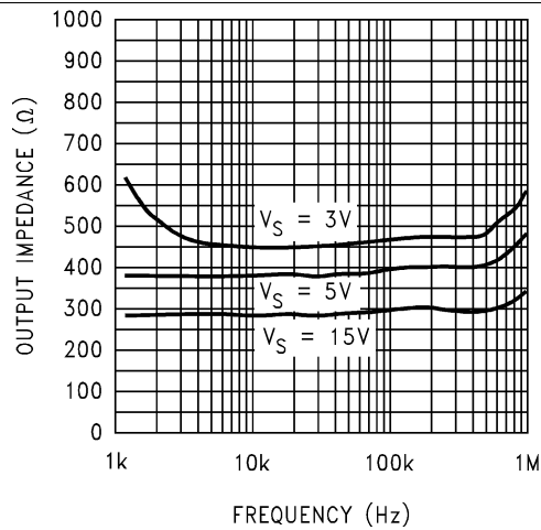
图 40. 输出阻抗与频率间的关系
