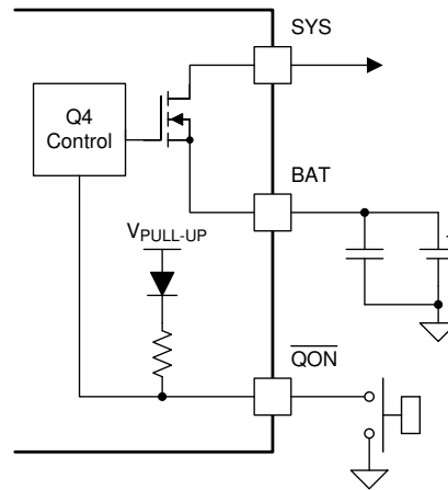
图 8-11. \overline{\text{QON}} Circuit
