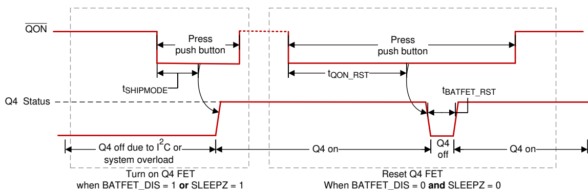
图 8-10. \overline{QON} Timing
