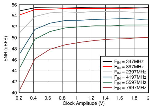
图 6-81. DES Mode: SNR vs Clock Amplitude
