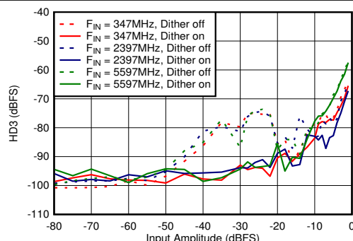
图 6-64. DES Mode: HD3 vs Input Amplitude and Dither
