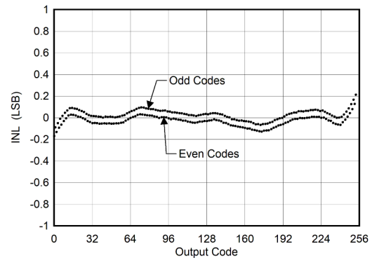
图 6-4. INL vs ADC Code
