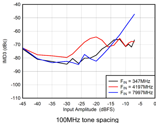
图 6-101. DES Mode: IMD3 vs Input Amplitude
