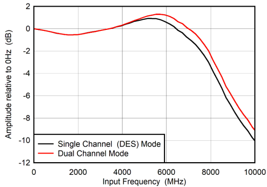
图 6-1. Input Amplitude vs Input Frequency
