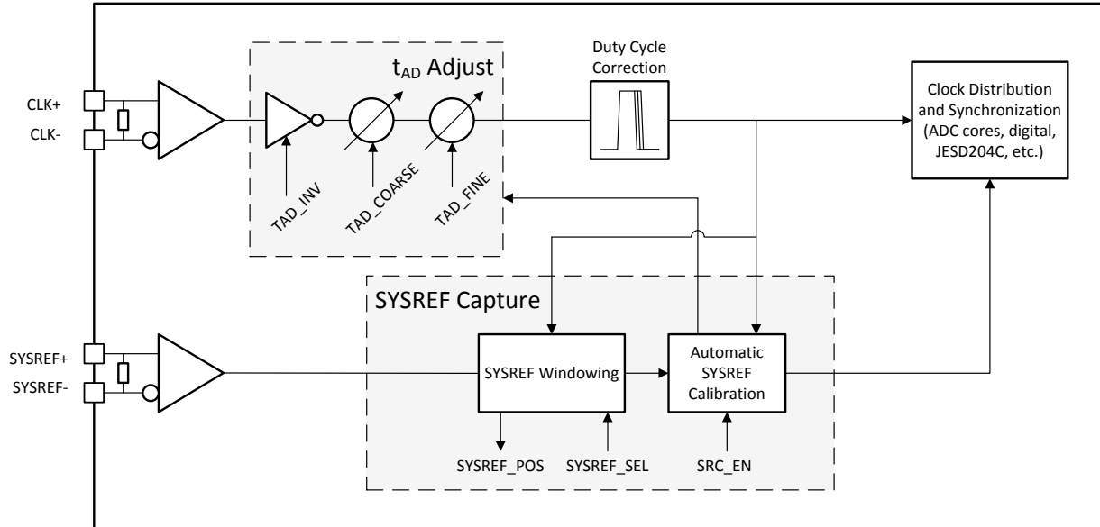
图 7-2. Clocking Subsystem
