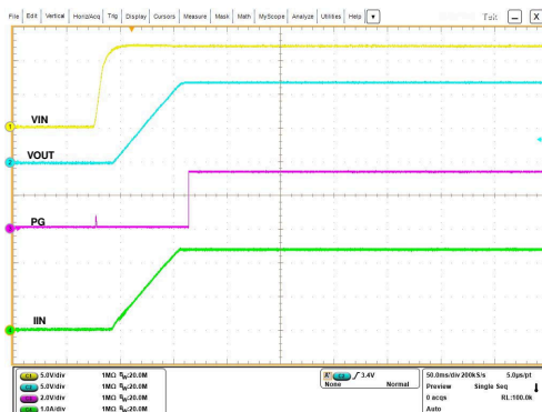
图 7-40. Input Hot-Plug
