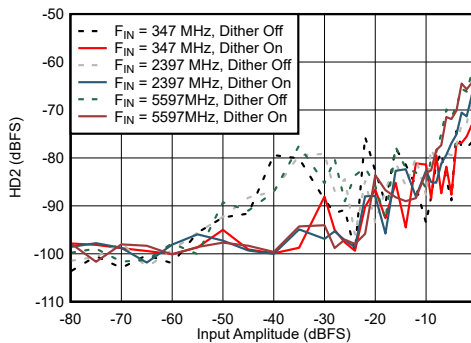
图 7-60. DES Mode: HD2 vs Input Amplitude and Dither
