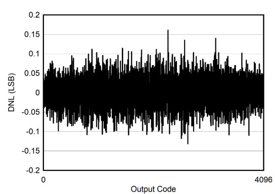
图 7-6. DNL vs ADC Code
