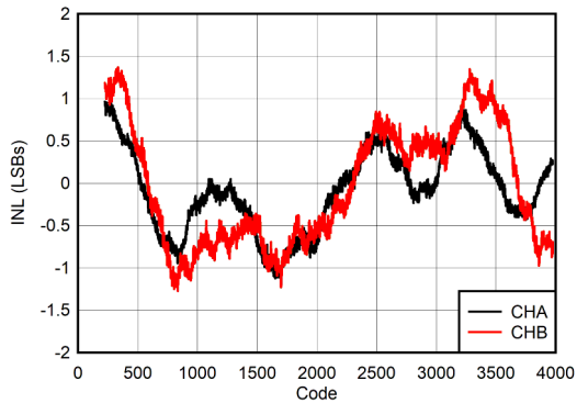
图 7-7. INL vs ADC Code
