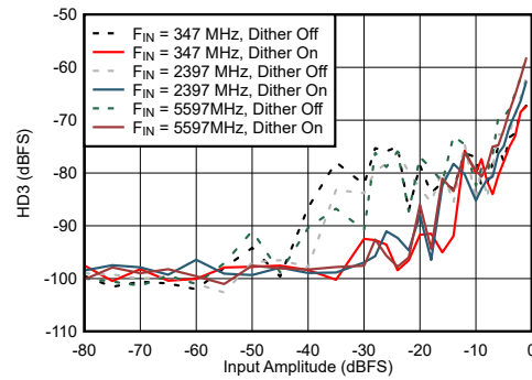
图 7-62. DES Mode: HD3 vs Input Amplitude and Dither
