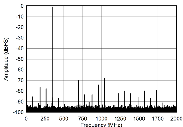
图 9-3. FFT for 347 MHz Input Signal, 4 GSPS, JMODE3
