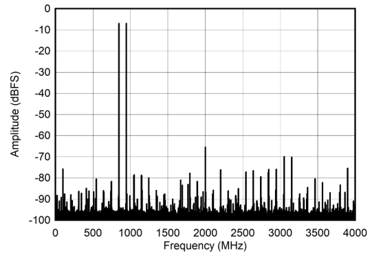
图 7-14. DES Mode: Two Tone FFT at 897 MHz
