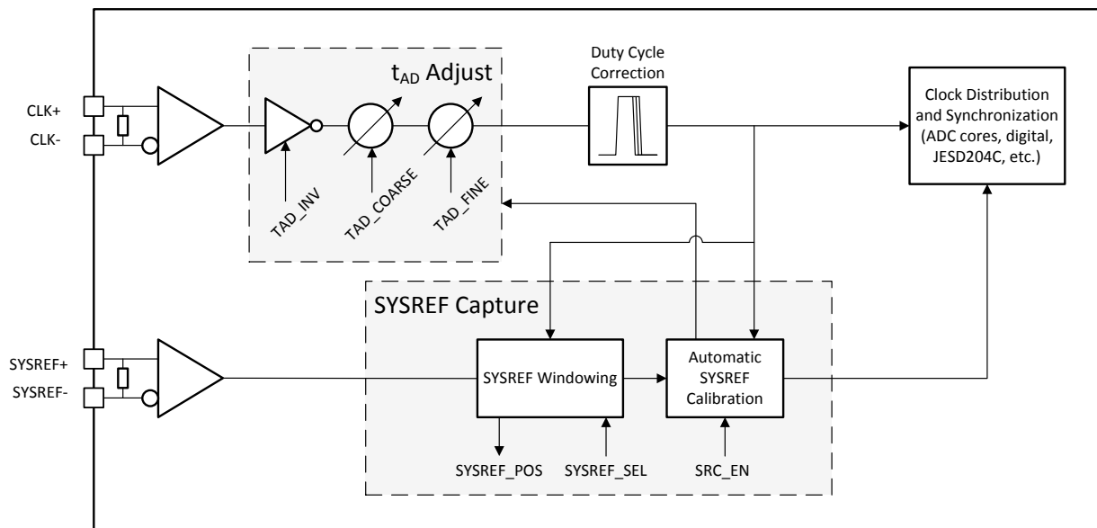
图 8-2. Clocking Subsystem
