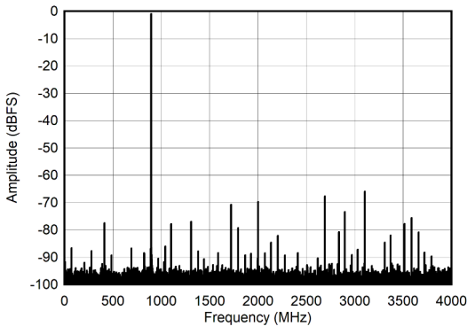
图 7-9. DES Mode: Single Tone FFT at 897 MHz
