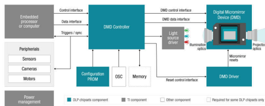
图 1. 1080p 全高清芯片组设计
