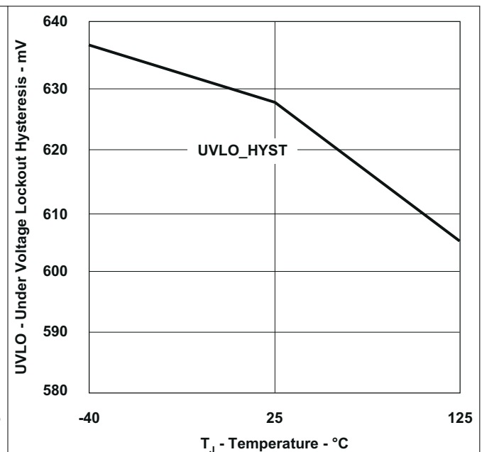
图 6-4. UVLO Hysteresis vs Temperature
