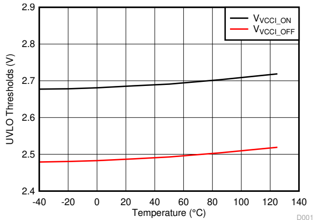
图 5-9. VCCI UVLO Threshold Voltage
