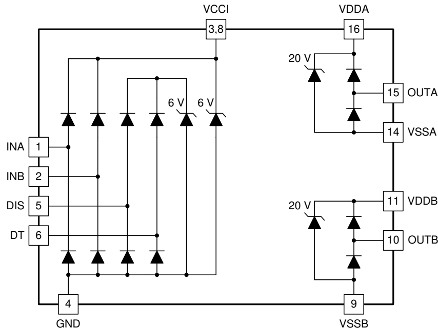
图 7-3. ESD Structure
