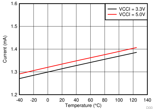
图 5-3. VCCI Quiescent Current
