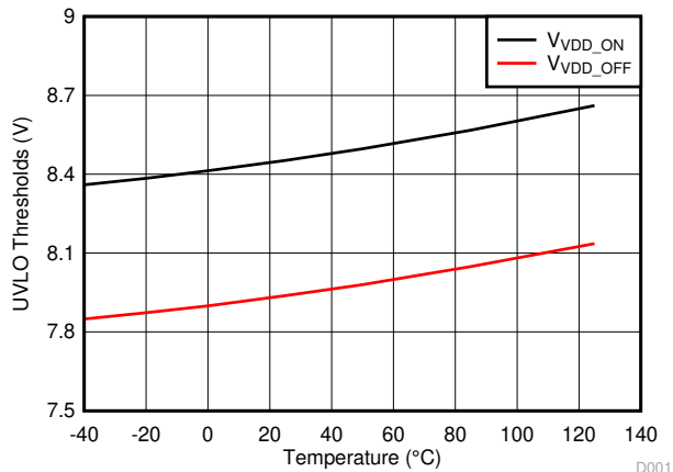
图 5-11. VDD UVLO Threshold Voltage
