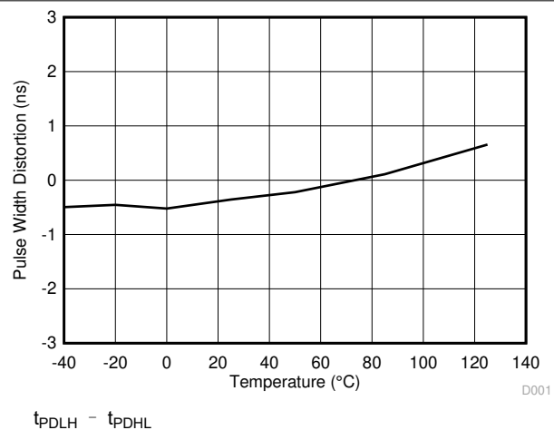
图 5-18. Pulse Width Distortion
