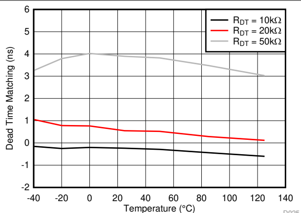
图 5-24. Dead Time Matching
