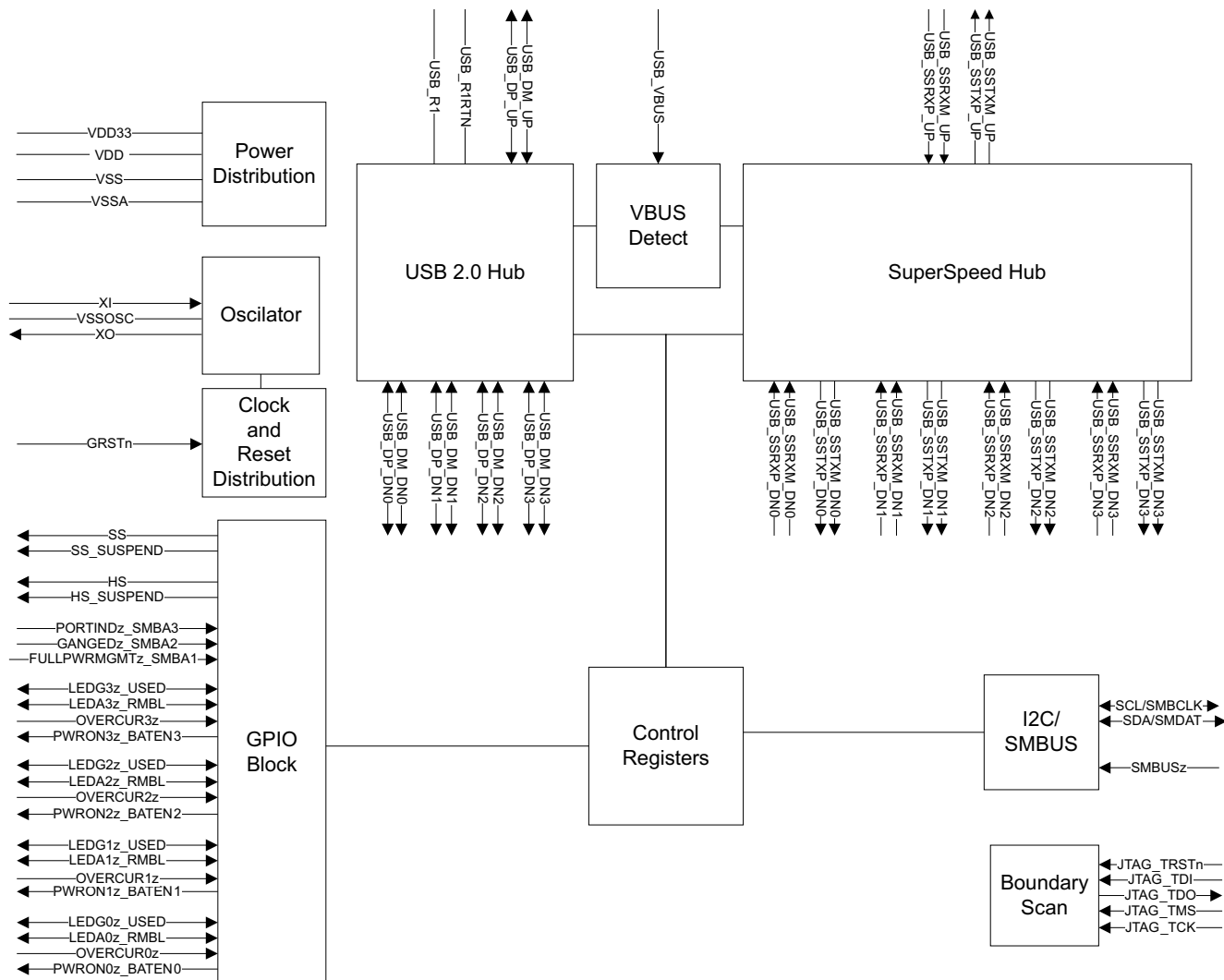
功能方框图
