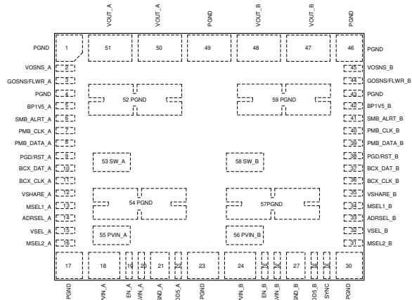
图 4-1. 59-Pin QFM-MOW Package (Top View)
