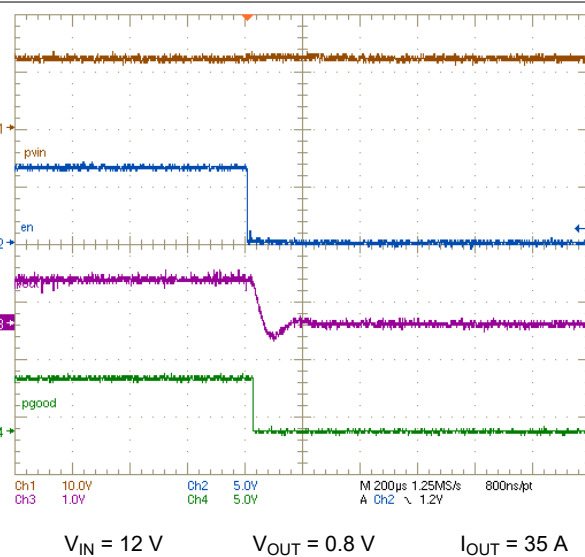
图 7-6. Shutdown from CNTL
