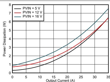
图 7-4. Power Dissipation
