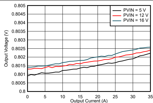
图 7-2. Load Regulation
