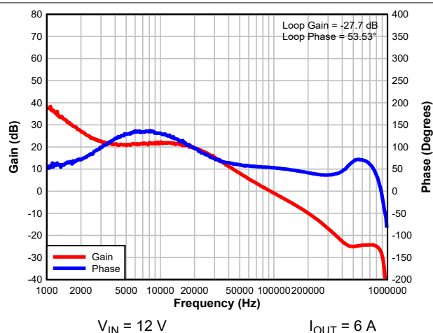
图 7-7. Bode Plot
