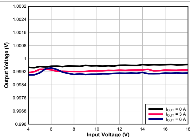
图 7-6. Line Regulation
