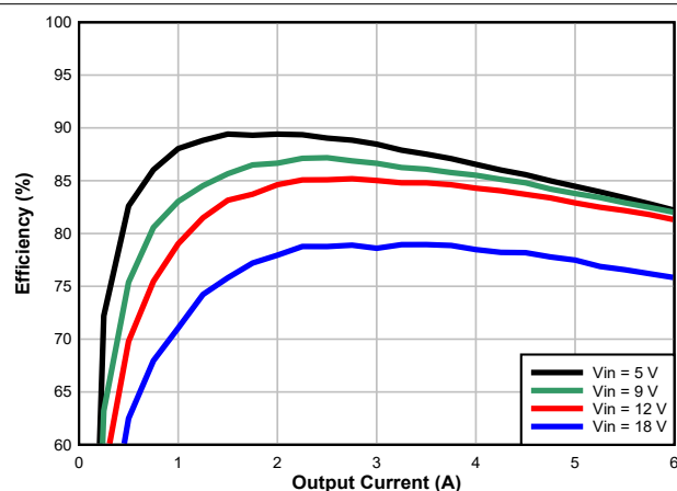
图 7-4. Efficiency
