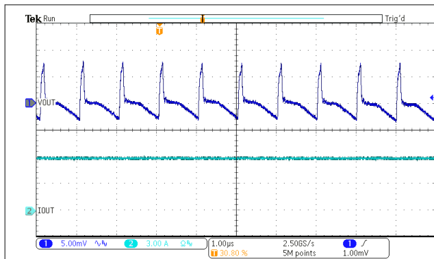
图 7-16. Output Ripple – 6-A Load
