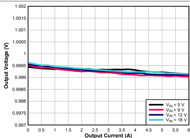
图 7-5. Load Regulation
