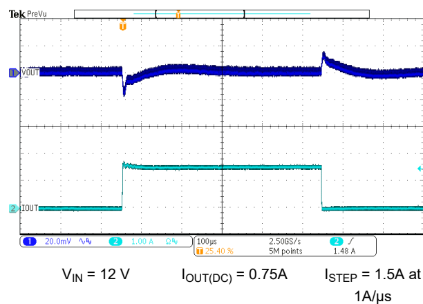
图 7-8. Load Transient
