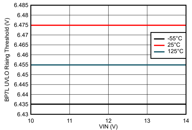
图 7-24. BP7L UVLO Rising Threshold vs VIN Voltage
