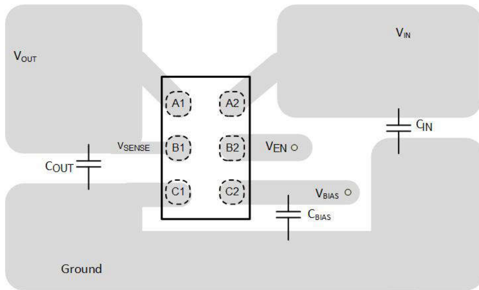
图 8-6. Recommended Layout (YBK Package)
