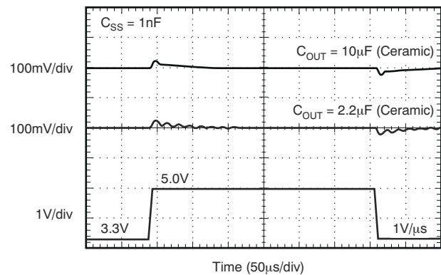
图 8-12. V_{\text{BIAS}} Line Transient
