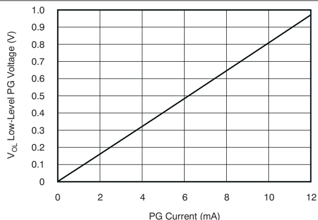
图 6-16. 低电平 PG 电压与电流间的关系
