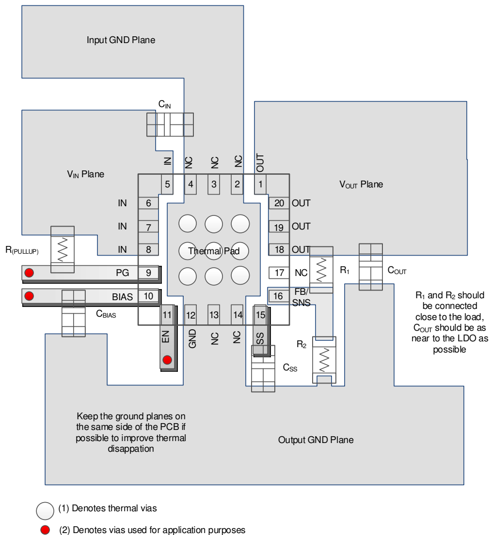
图 8-16. Layout Example (RGW Package)
