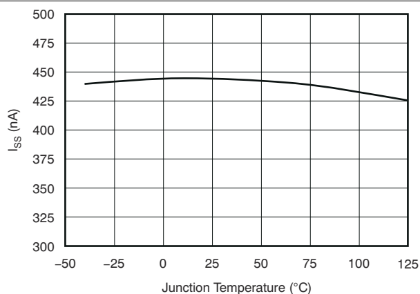
图 6-15. 软启动充电电流 ( I_{SS} ) 与温度 ( T_J ) 间的关系
