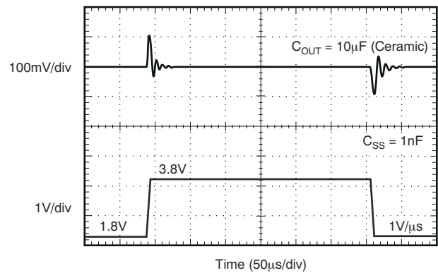
图 8-4. V_{IN} Line Transient
