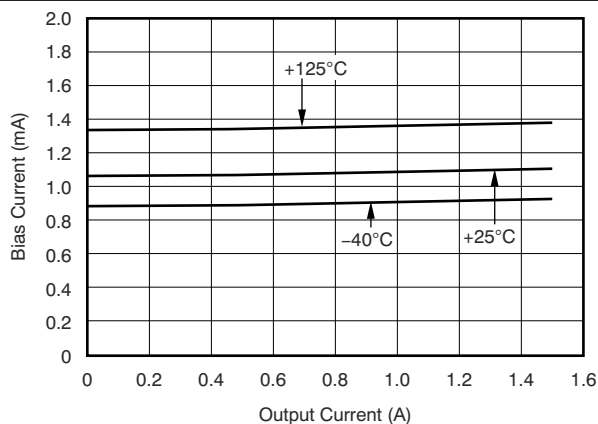
图 6-13. BIAS 引脚电流与输出电流和温度 ( T_J ) 间的关系
