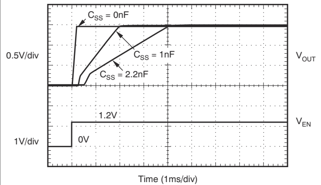
图 8-6. Turn-On Response
