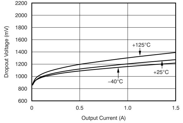
图 6-8. V_{BIAS} 压降电压与 I_{OUT} 和温度 ( T_J ) 间的关系
