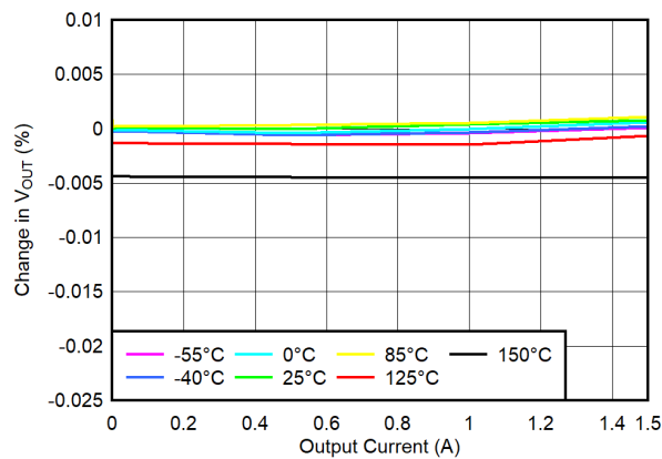
图 6-25. Load Regulation
