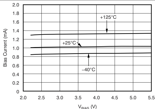
图 6-14. BIAS 引脚电流与 V_{BIAS} 和温度 ( T_J ) 间的关系
