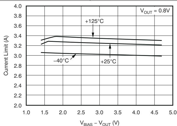
图 6-17. 电流限值与 (V_{BIAS} - V_{OUT}) 间的关系
