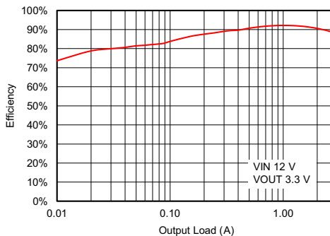
效率与输出负载之间的关系
