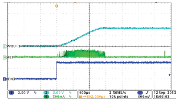
图 8-7. Buck3, Soft-Start With No Load
