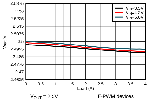
图 8-18. Load Regulation
