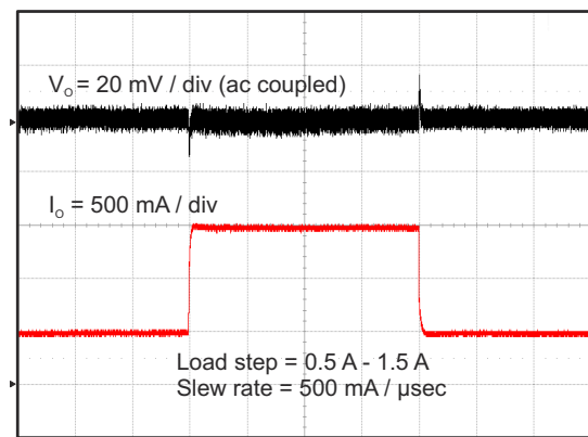
图 8-11. Tps562200 Transient Response
