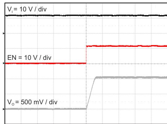
图 8-13. Tps562200 Start Up Relative to En
