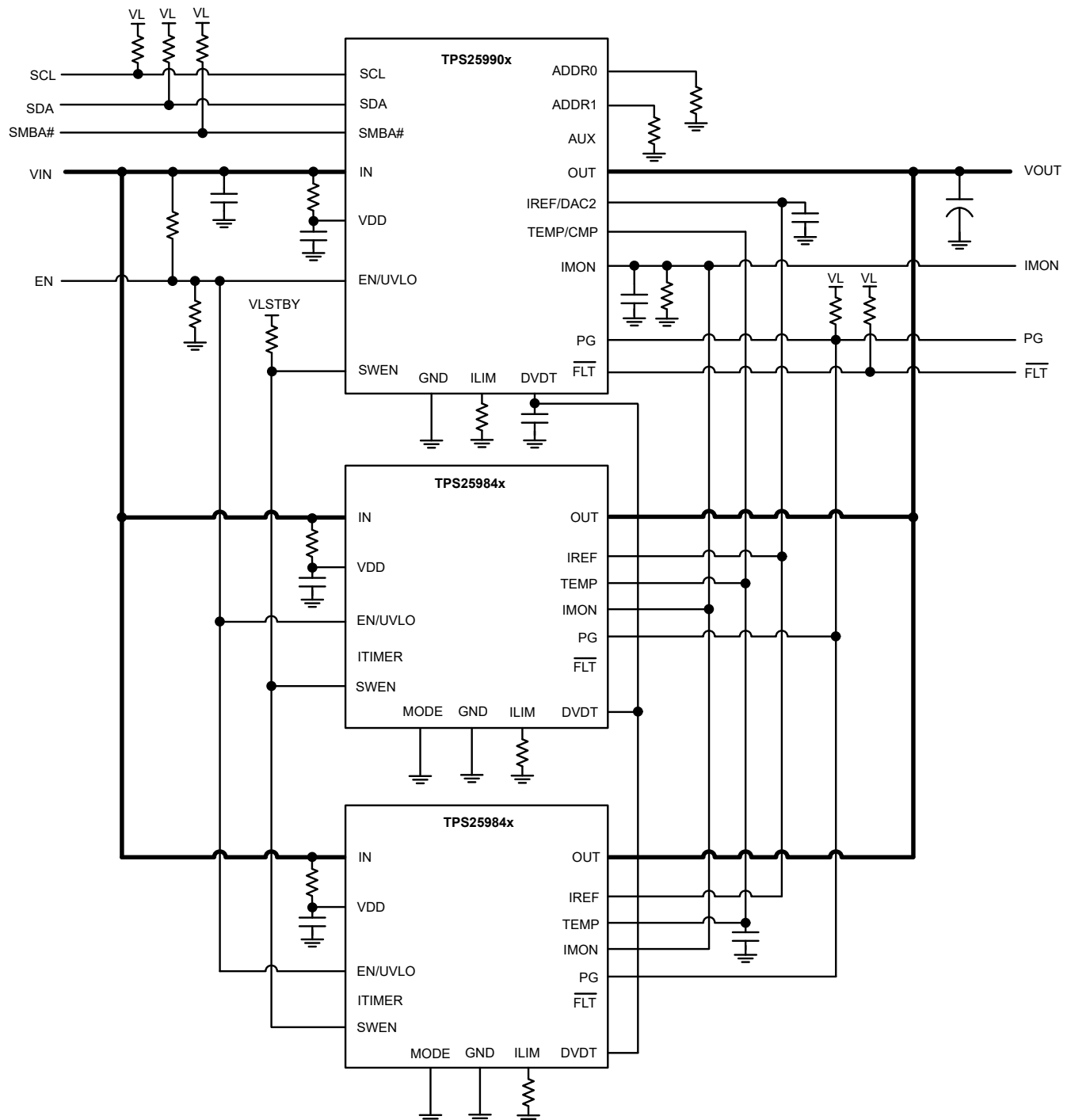
图 9-3. TPS25990x 连接到 TPS25984x 以支持更高的电流并带有 PMBus®
