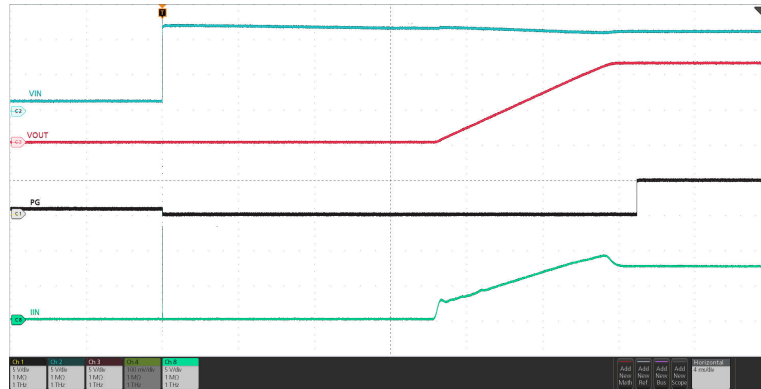
图 8-2. Insertion Delay
