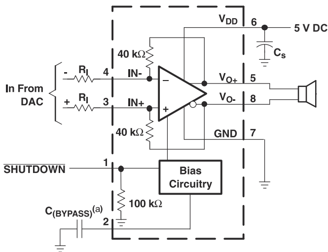
应用电路
