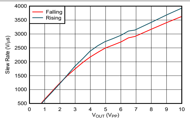
图 7-14. Slew Rate vs Output Voltage Step
