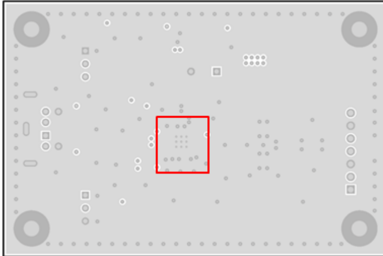
Figure 21. Bottom Layer
