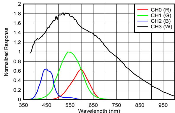
归一化光谱响应
