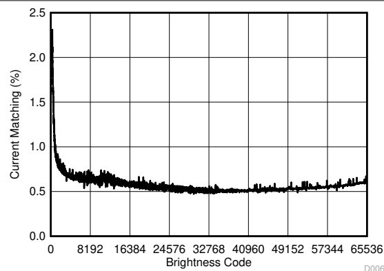
图 6-7. Current Matching
