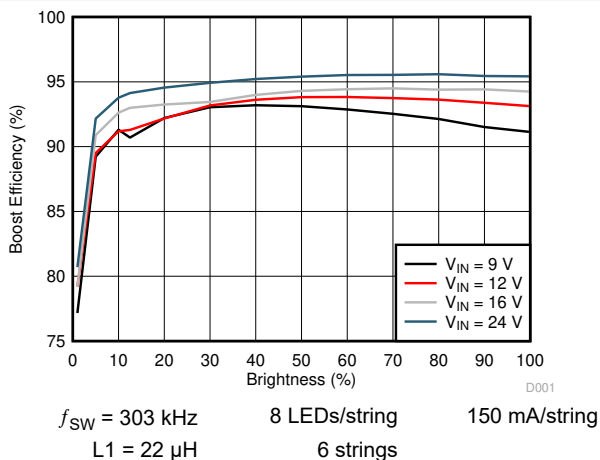
图 6-2. Boost Efficiency
