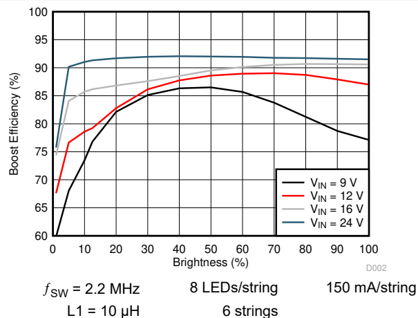
图 6-3. Boost Efficiency
