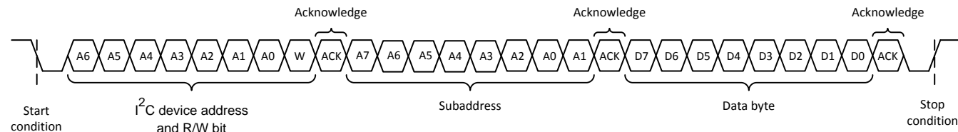
图 24. Single-Byte Write Transfer
