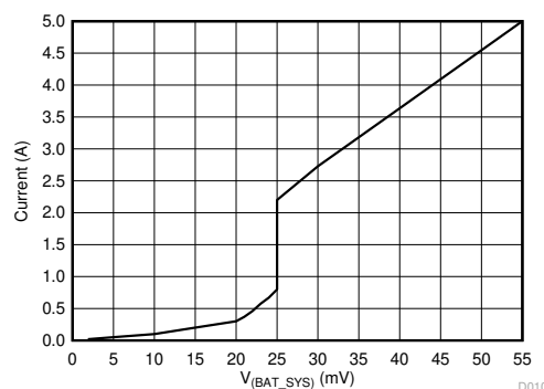
图 8-4. BATFET V-I Curve
