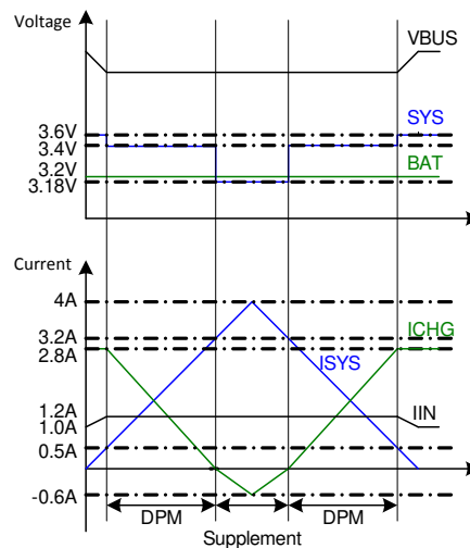
图 8-3. DPM Response
