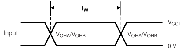
图 8-4. 脉冲持续时间 (推挽)
