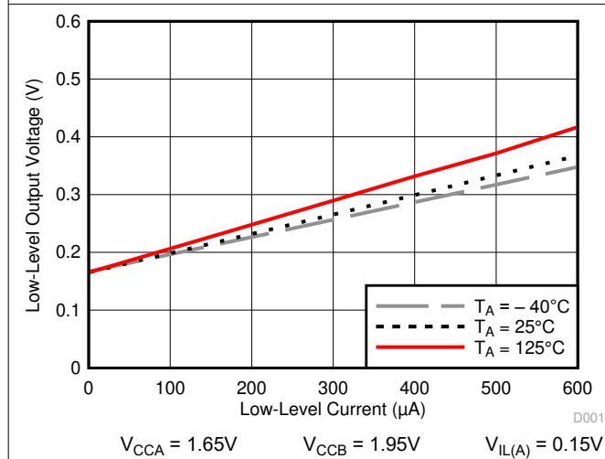
图 7-3. 低电平输出电压 ( V_{OL(Bx)} ) 与低电平电流 ( I_{OL(Bx)} ) 间的关系
