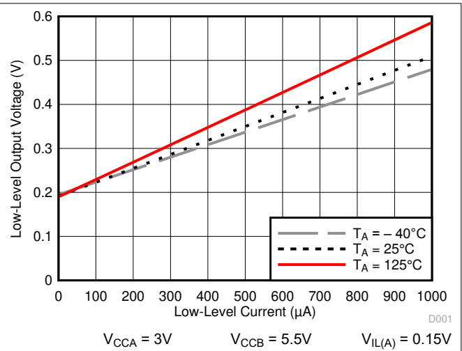
图 7-2. 低电平输出电压 ( V_{OL(Bx)} ) 与低电平电流 ( I_{OL(Bx)} ) 间的关系
