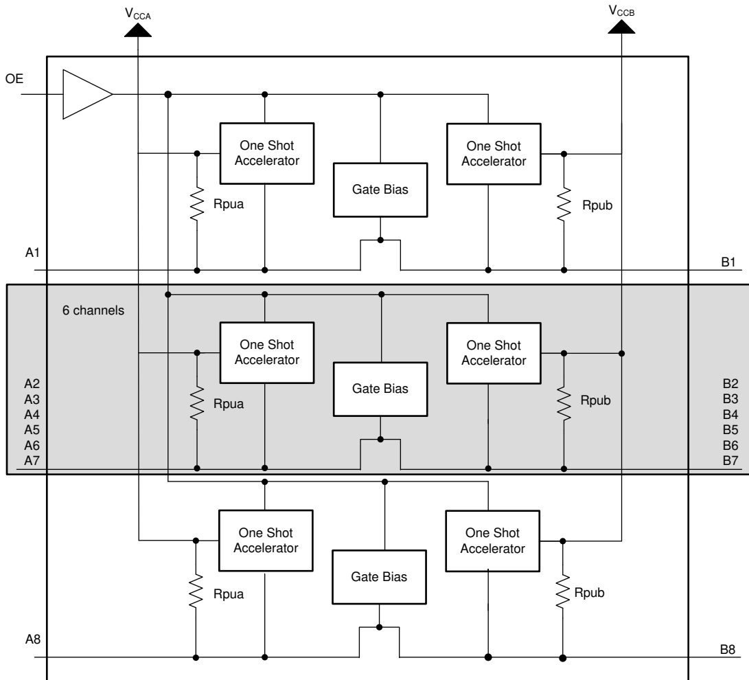
图 9-1. 功能方框图
