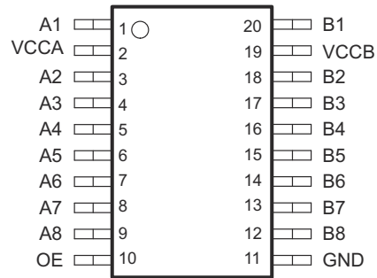
图 5-1. PW 封装 20 引脚 TSSOP (顶视图)
