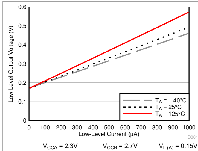
图 7-1. 低电平输出电压 ( V_{OL(Bx)} ) 与低电平电流 ( I_{OL(Bx)} ) 间的关系
