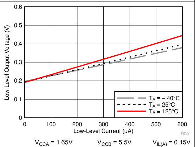
图 7-4. 低电平输出电压 ( V_{OL(Bx)} ) 与低电平电流 ( I_{OL(Bx)} ) 间的关系
