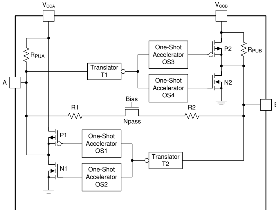
图 9-2. TXS0108E-Q1 单元的架构
