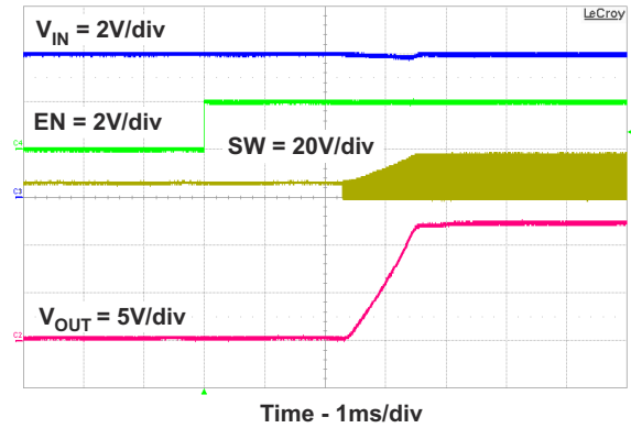
图 9-15. Output Voltage Soft-Start
