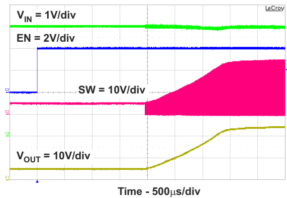
图 9-8. Start Up
