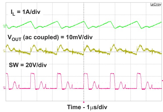
图 9-6. DCM PWM Operation
