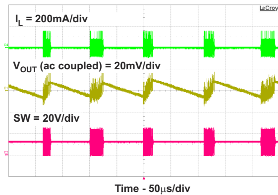
图 9-7. Pulse Skipping
