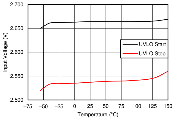
图 7-9. Input Voltage UVLO vs Temperature
