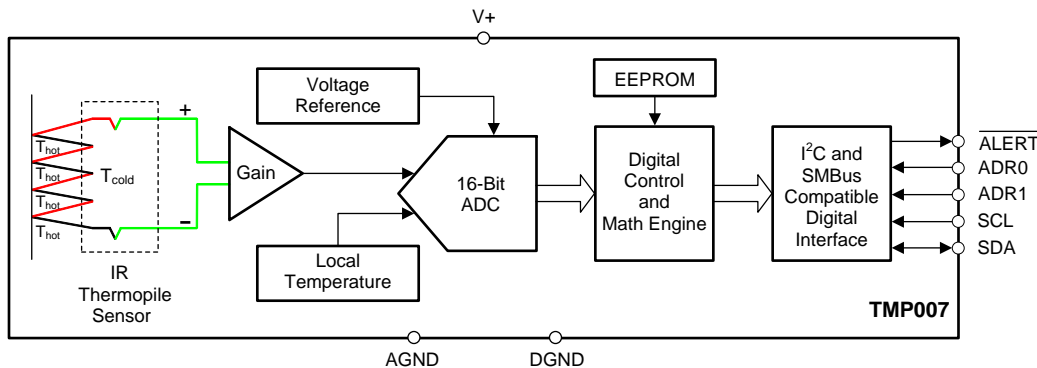
功能方框图
