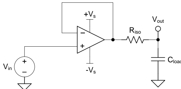
图 62. 使用 OPA192 扩展容性负载驱动
