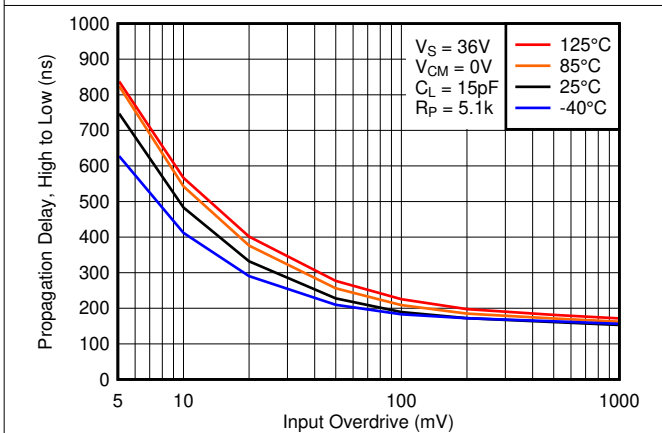
图 6-34. 高电平至低电平传播延迟与输入过驱电压之间的关系, 36V
