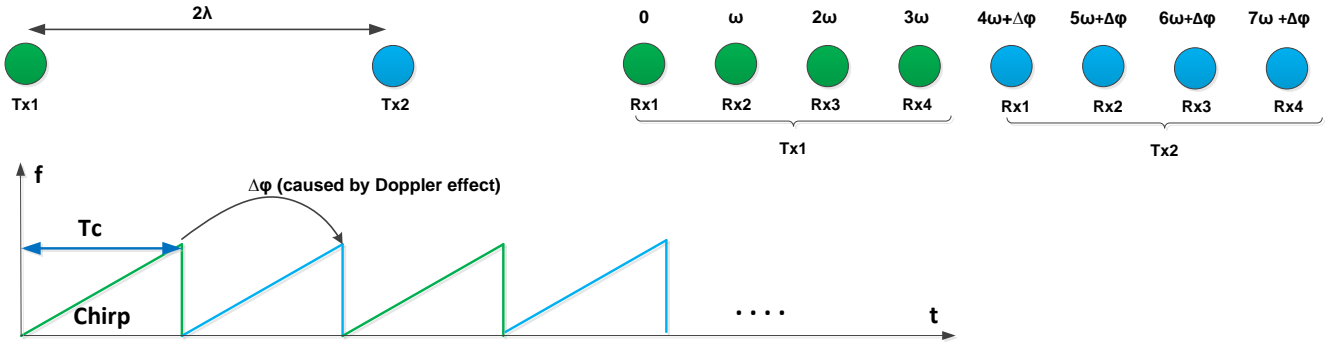
图 7. TDM MIMO 相偏补偿原理图
